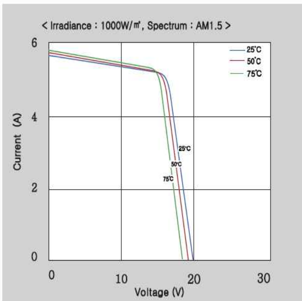
< Irradiance : 1000W/m 2 , Spectrum : AM1.5 >
