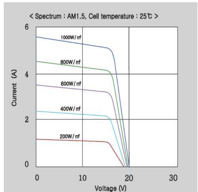
< Spectrum : AM1.5, Cell temperature : 25°C >
